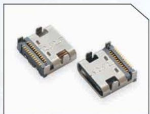
板上双排SMT母座
